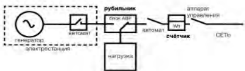
Схема подключения автономного источника питания с использованием автоматики включения резерва электропитания:
